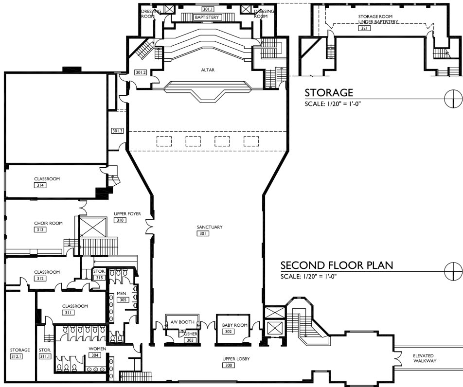
二層平面圖
