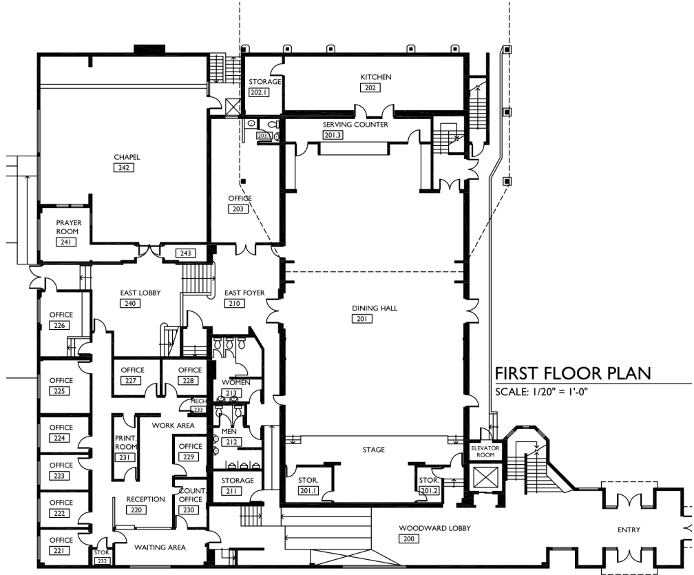
一層平面圖
