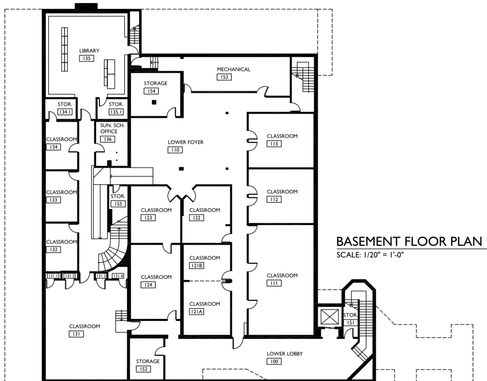
地庫平面圖
